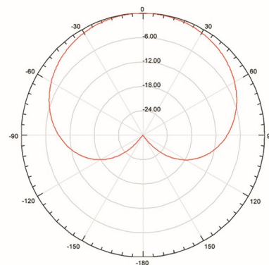
1205MHz-1278MHz
